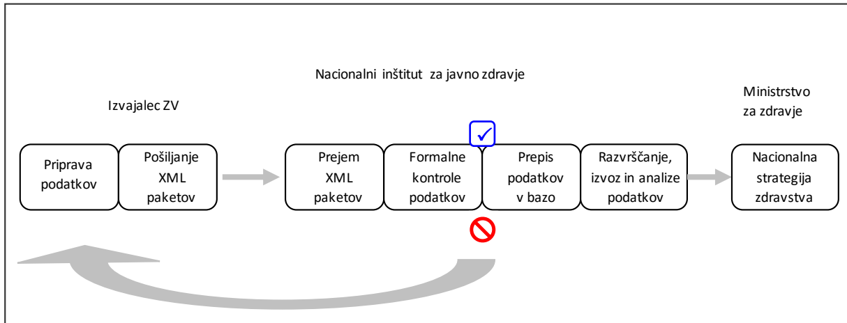
Slika 1: Aplikacija ePrenosi
